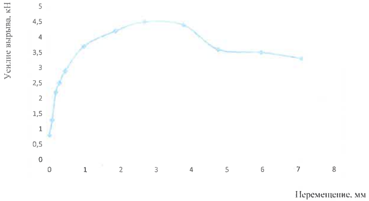
Рис. 11 (Точка № 11) Максимальное усилие 4,5 кН
