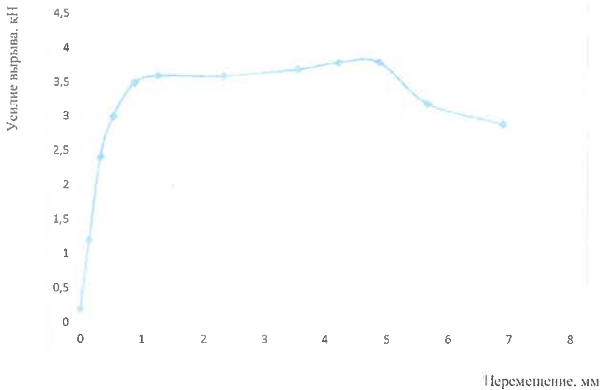
Рис. 12 (Точка № 12) Максимальное усилие 3,8 кН
